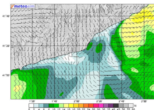
14:00 h dissabte (Model Mass, pas malla 2.5 km)
