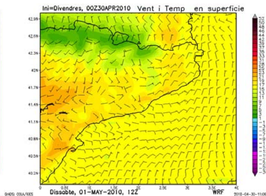
14:00 h (Model WRF, pas malla 9 km)
